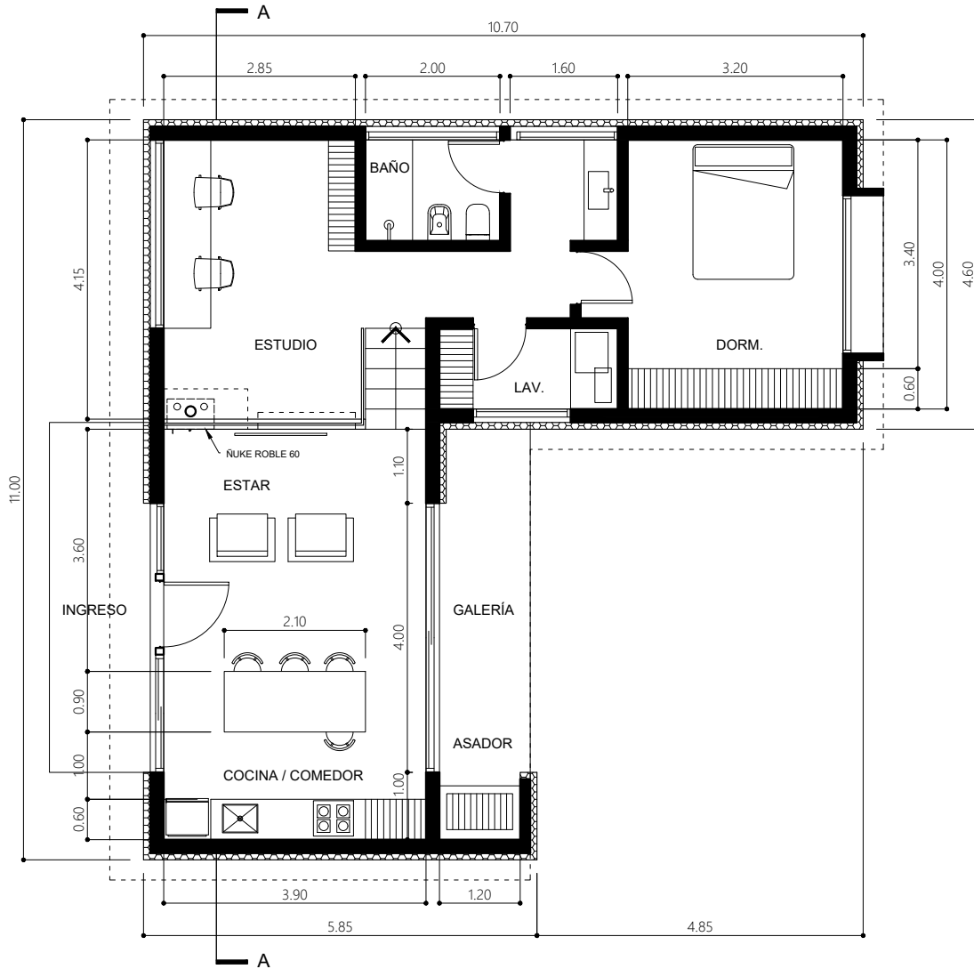
PLANTA GENERAL 1:100
