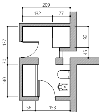
PLANO EXISTENTE
